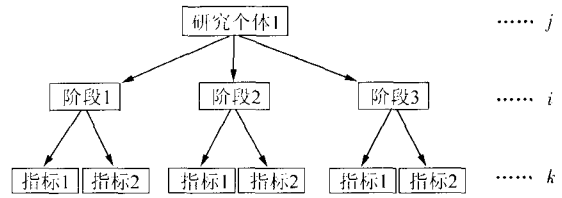
图 1 两指标三水平层次结构示意图
